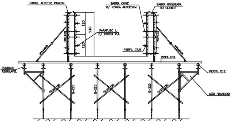
CORTE A-A
