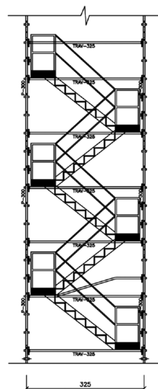
VISTA LATERAL
